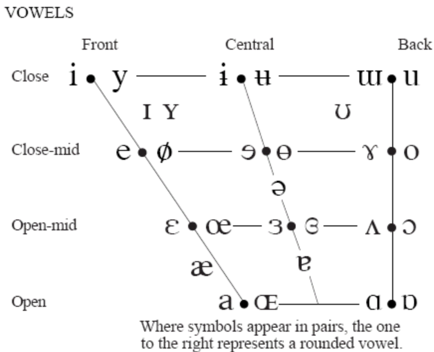
Slika 1. Vokalski trapez prema IPA-i ; ako su simboli prikazani u paru, onaj koji se nalazi na desnoj strani simbolizira zaokruženi vokal (IPA, 2005)
