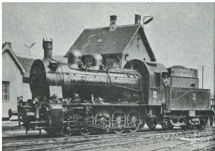
Lokomotiva serije JŽ 35 (DRB 57), 510 kW Proizvedena 1919. godine
