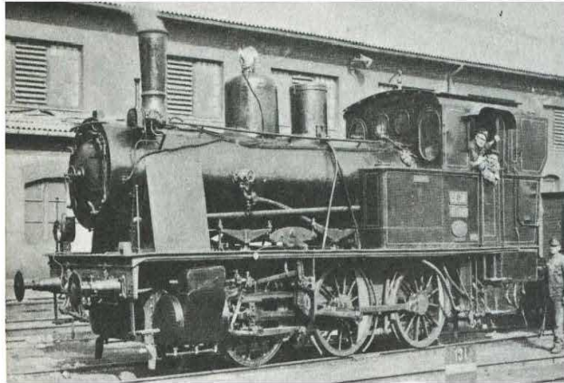
Lokomotiva JŽ 61 (SDŽ 2000), 210 kW Proizvedena 1918. godine
