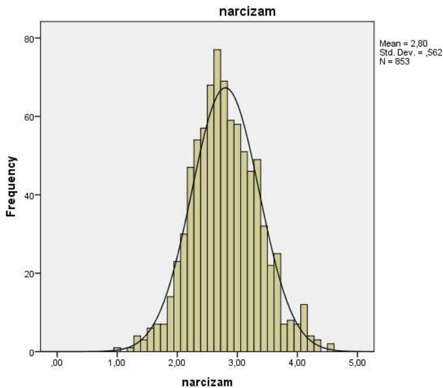
Slika 4. Grafički prikaz distribucije rezultata na ljestvici narcizma za djevojke
