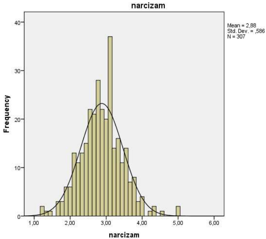
Slika 3. Grafički prikaz distribucije rezultata na ljestvici narcizma za mladiće
