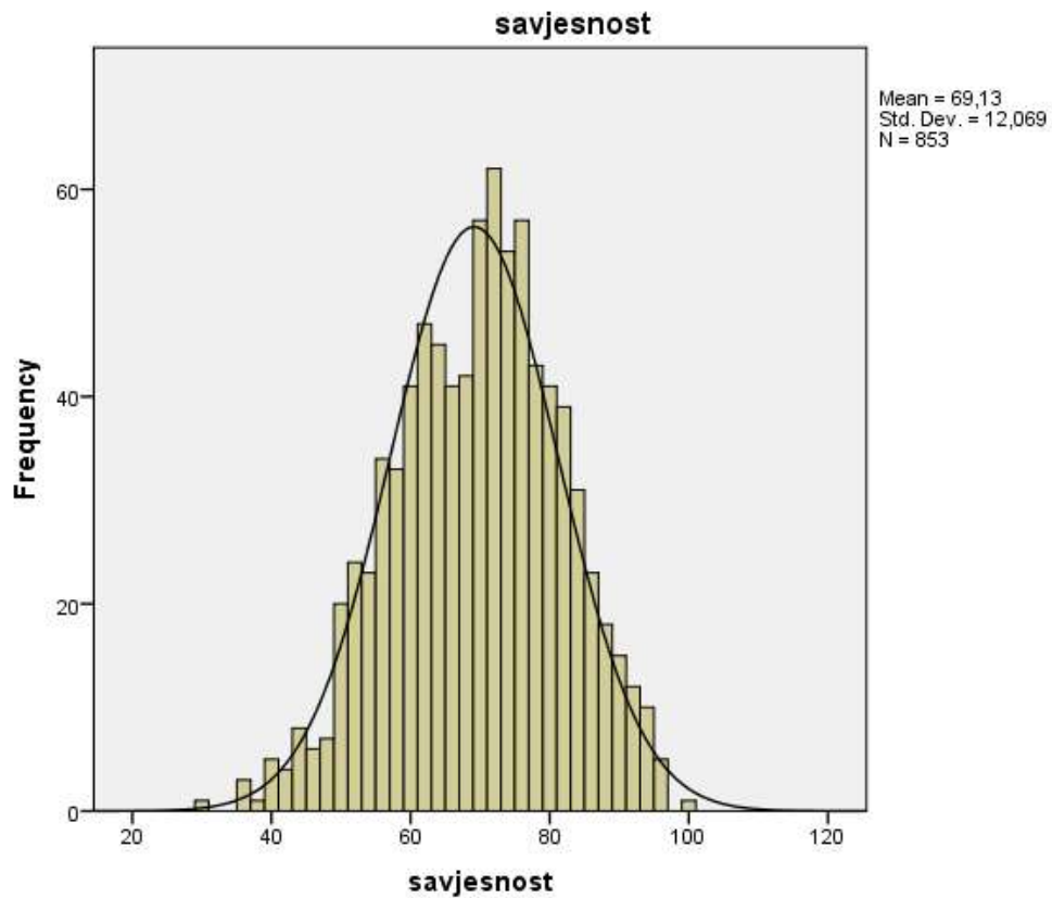
Slika 16. Grafički prikaz distribucije rezultata na ljestvici savjesnosti za djevojke
