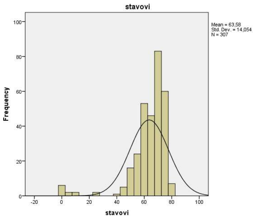
Slika 19. Grafički prikaz distribucije rezultata na ljestvici prepoznavanja nasilja u vezama mladih za mladiće
