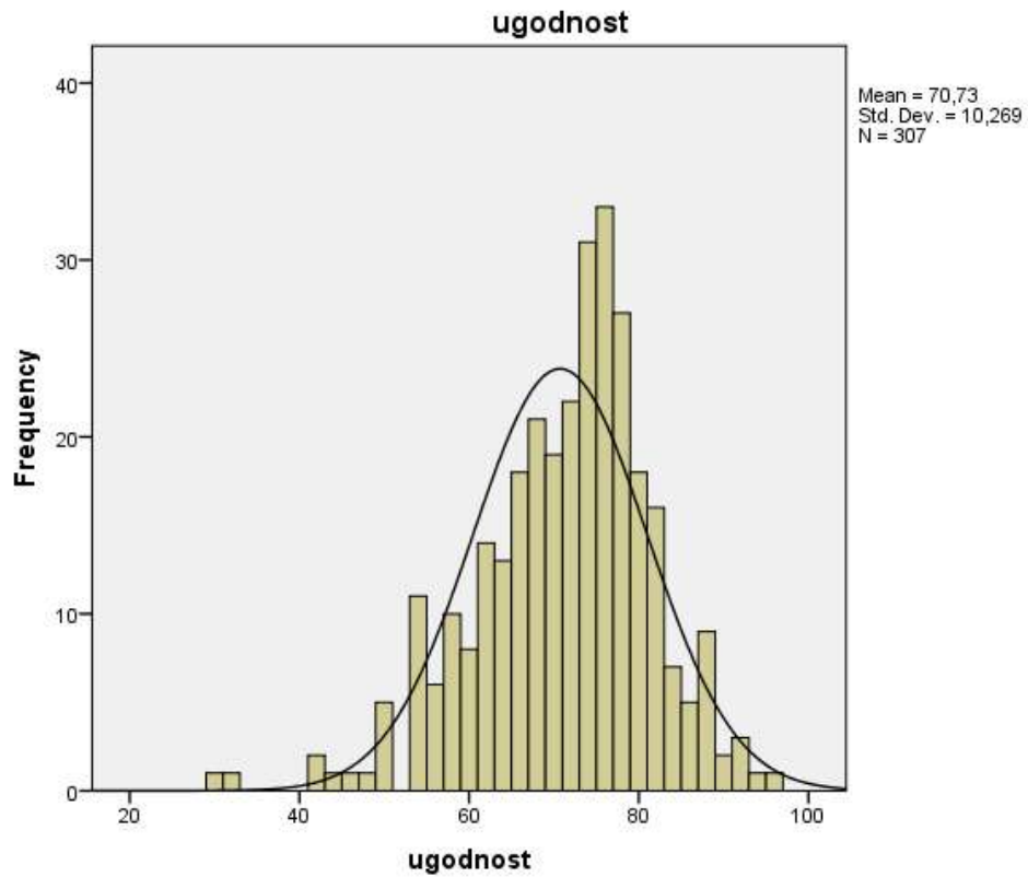
Slika 13. Grafički prikaz distribucije rezultata na ljestvici ugodnosti za mladiće
