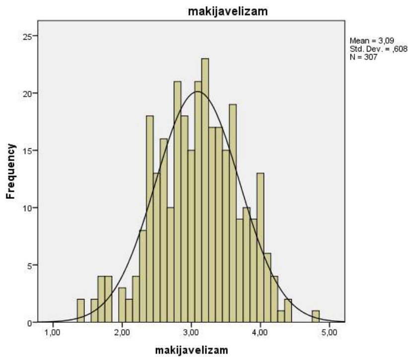
Slika 1. Grafički prikaz distribucije rezultata na ljestvici makijavelizma za mladiće
