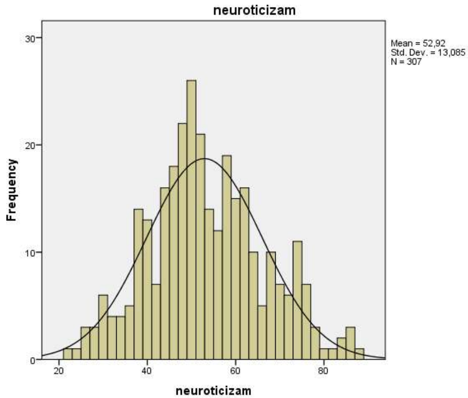
Slika 7. Grafički prikaz distribucije rezultata na ljestvici neuroticizma za mladiće
