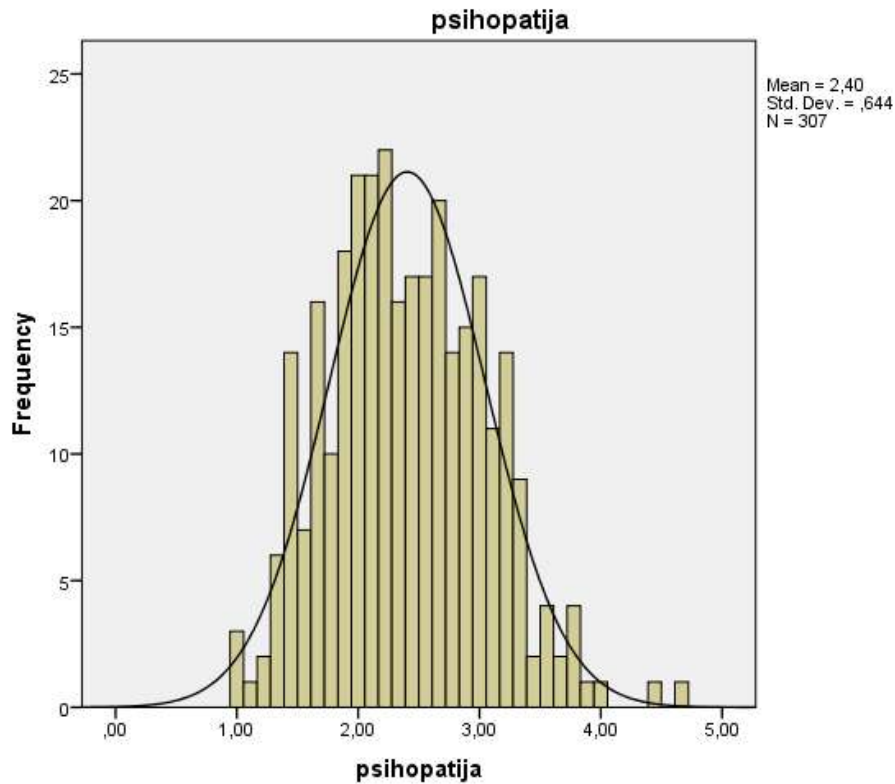
Slika 5. Grafički prikaz distribucije rezultata na ljestvici psihopatije za mladiće
