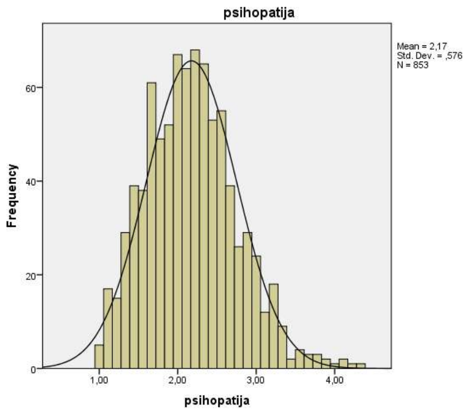
Slika 6. Grafički prikaz distribucije rezultata na ljestvici psihopatije za djevojke
