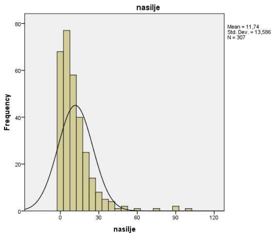
Slika 17. Grafički prikaz distribucije rezultata na ljestvici počinjenja nasilja u vezama mladih za mladiće
