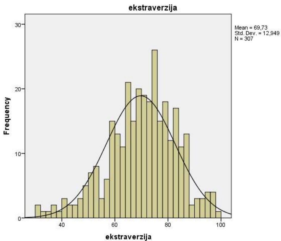
Slika 9. Grafički prikaz distribucije rezultata na ljestvici ekstraverzije za mladiće
