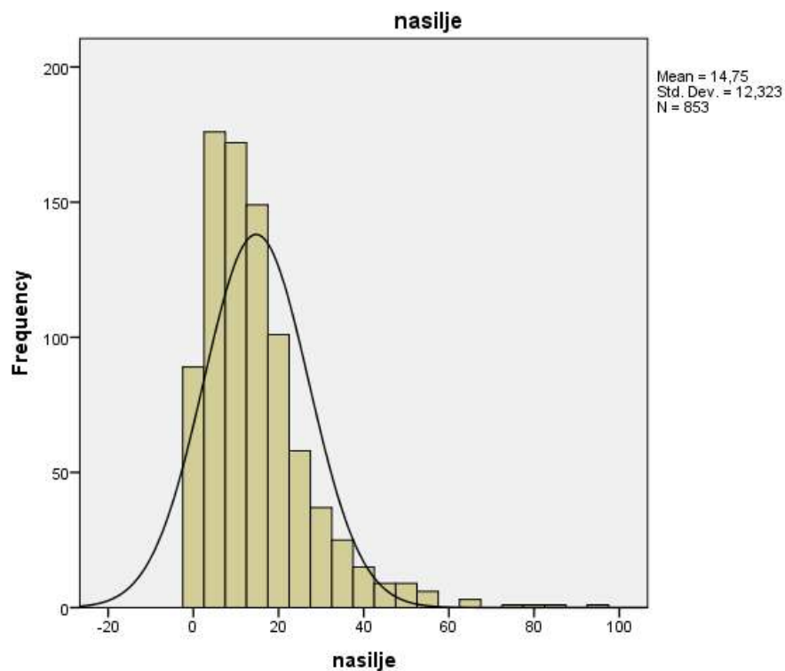
Slika 18. Grafički prikaz distribucije rezultata na ljestvici počinjenja nasilja u vezama mladih za djevojke
