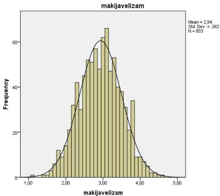
Slika 2. Grafički prikaz distribucije rezultata na ljestvici makijavelizma za djevojke
