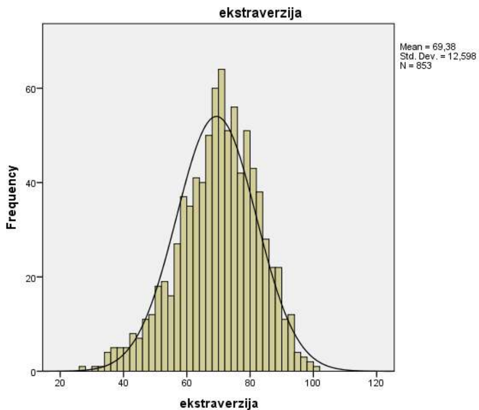
Slika 10. Grafički prikaz distribucije rezultata na ljestvici ekstraverzije za djevojke
