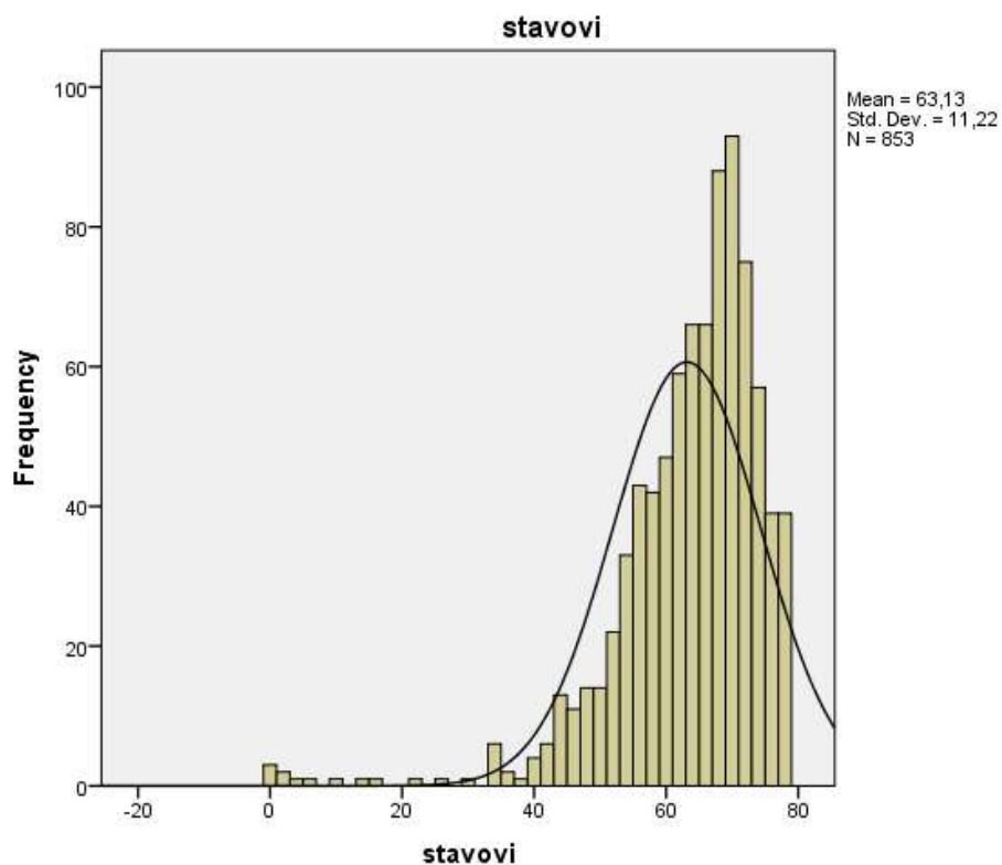
Slika 20. Grafički prikaz distribucije rezultata na ljestvici prepoznavanja nasilja u vezama mladih za djevojke
