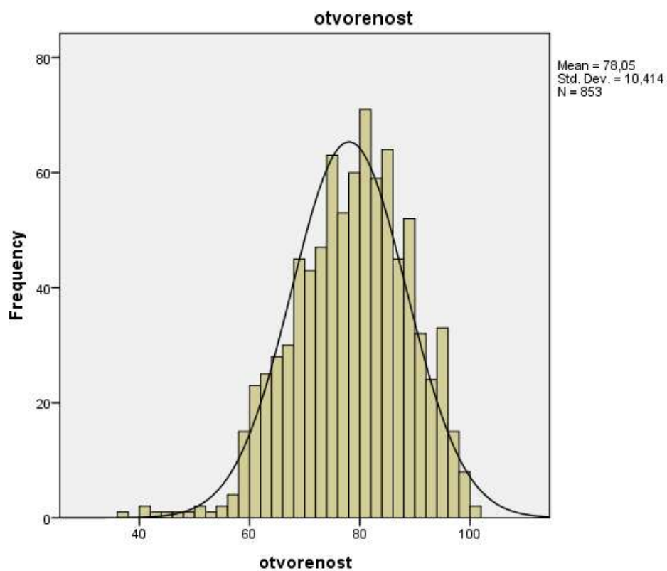
Slika 12. Grafički prikaz distribucije rezultata na ljestvici otvorenosti iskustvu za djevojke
