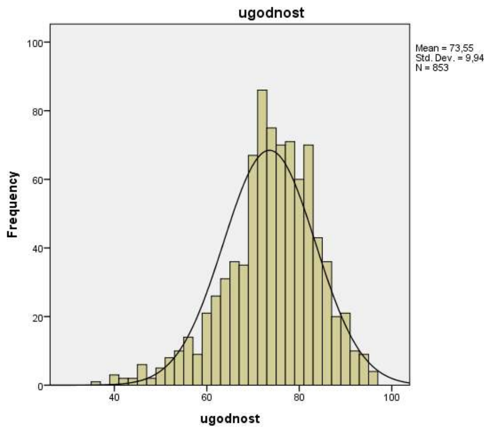
Slika 14. Grafički prikaz distribucije rezultata na ljestvici ugodnosti za djevojke
