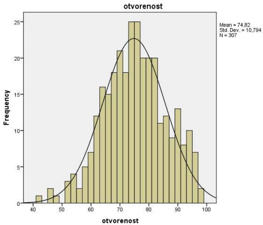
Slika 11. Grafički prikaz distribucije rezultata na ljestvici otvorenosti prema iskustvu za mladiće
