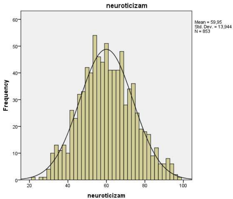
Slika 8. Grafički prikaz distribucije rezultata na ljestvici neuroticizma za djevojke
