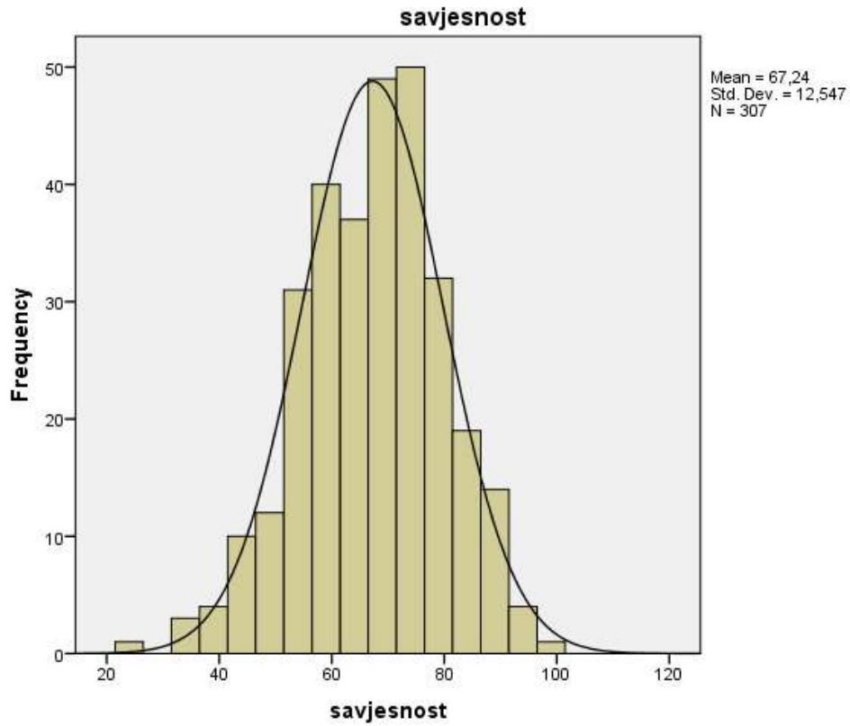
Slika 15. Grafički prikaz distribucije rezultata na ljestvici savjesnosti za mladiće
