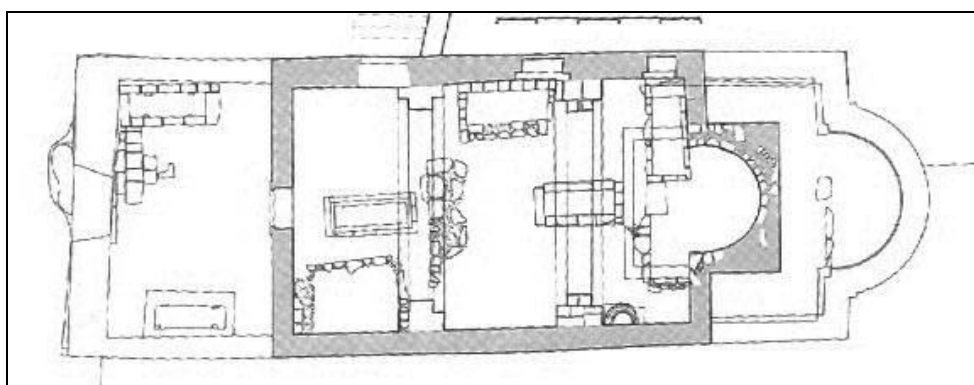
Sl. 18. Tlocrt crkve sv. Stjepana, predromanička faza, prema rezultatima istraživanja iz 1998. godine
