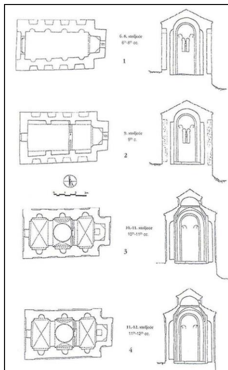
Sl. 24. Crkva Preobraženja Kristova (Sigurata), razvojne faze
