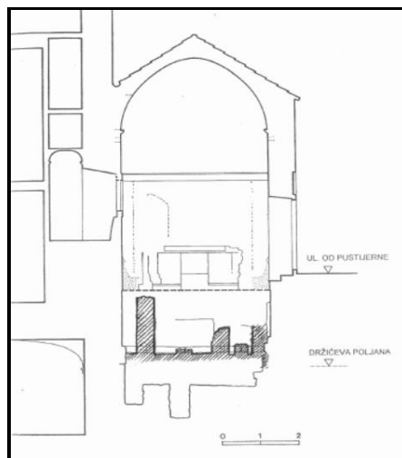
Sl. 27. Presjek crkve sv. Bartula s ostacima crkve sv. Kuzme i Damjana i ostacima ranije kule
