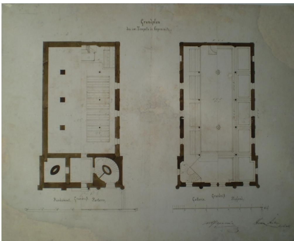
Slika 32.: (?) Popović, Hein Anton: „Grundplan des isr. Tempel in Koprivnitz“; tlocrti izraelitskog hrama u Koprivnici, bez datacije
