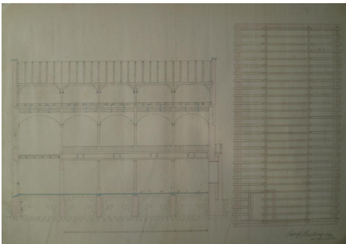
Slika 20.: Josef Heuberger: Uzdužni presjek, plan podnice krovništa, bez datacije
