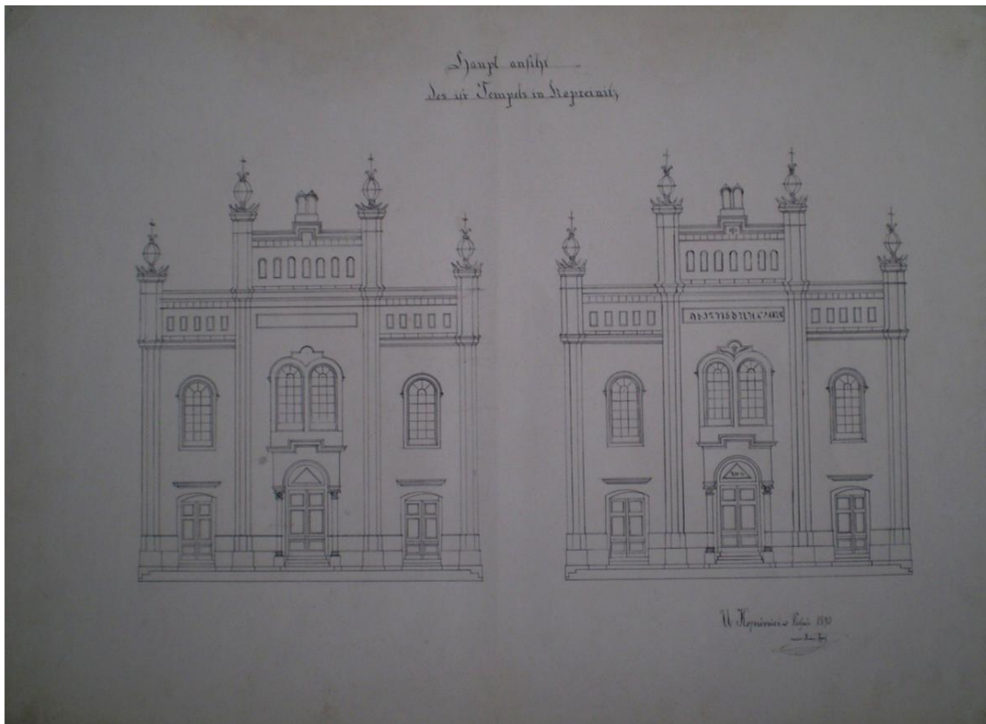
Slika 35.: Ivan Igrić :“ Haupt ansicht des isrl. Tempels in Koprivnitz“; Glavno pročelje izraelitičkog hrama u Koprivnici. U Koprivnici, 3. Veljače 1893.
