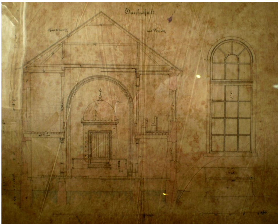
Slika 28.: Nepoznati arhitekt (moguće Popović i Hein): „Durchschnitt“; poprečni presjek, bez datacije
