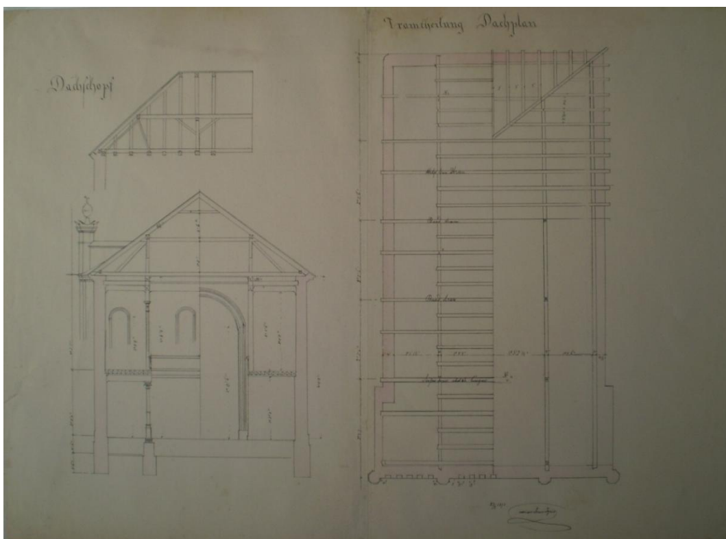
Slika 36.: Ivan Igrić: „Dachkopf, Tramtherlung Dachplan“ 25/3 1893; Presjek i plan krovišta, 25. ožujka 1893.
