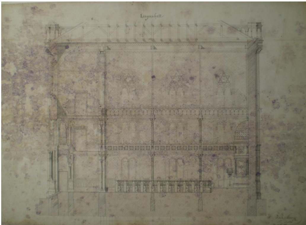
Slika 16.: Wilhem Stiassny: „Längenschnitt“, Wien, 22. Nov. 1867.; Uzdužni presjek, Beč, 22. studenog 1867.
