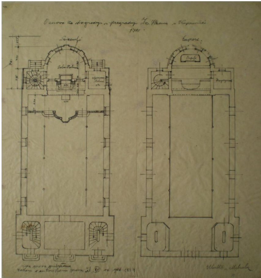
Slika 37.: Wutte Mikula (?): "Osnova za dogradnju i pregradnju Izr. Hrama u Koprivnici", bez datacije
