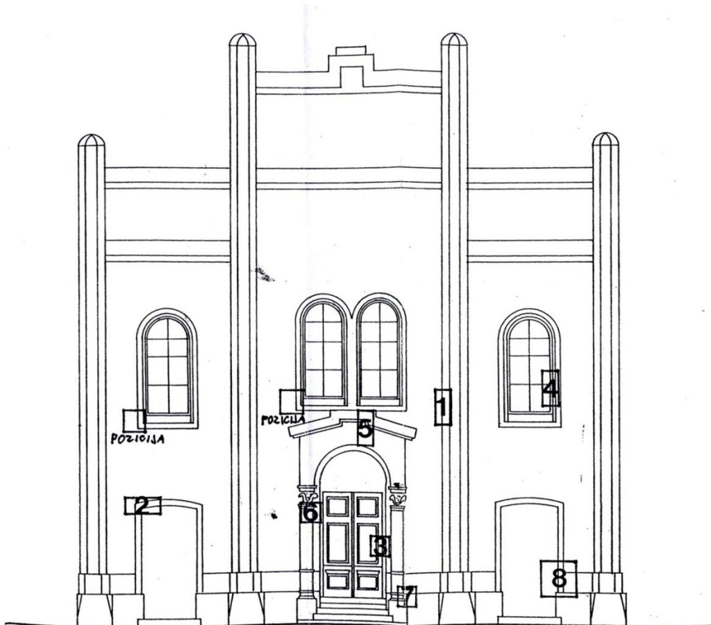
Slika 50.: Plan sondiranja fasade i nacrt obnove eksterijera
