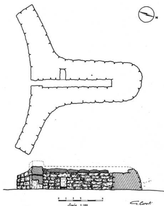
Slika 20. Plan i presjek megalitske grobnice na lokalitetu Sa Domu 'e s'Orku-Siddi
