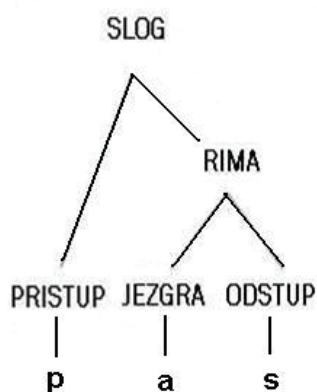
Slika 1. Struktura sloga
