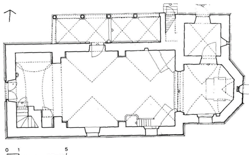
Slika 14. Tlocrt crkve Svete Marije Magdalene (Samaržija 1993:155)
